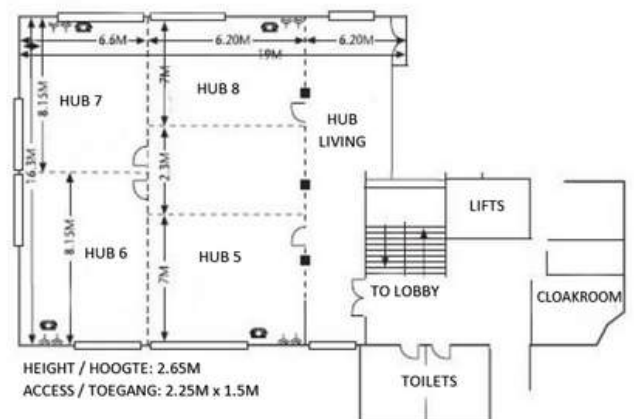
FIRST FLOOR / 1E VERDIEPING
